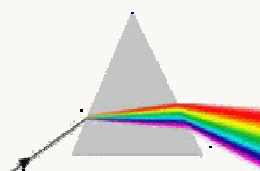
色散
